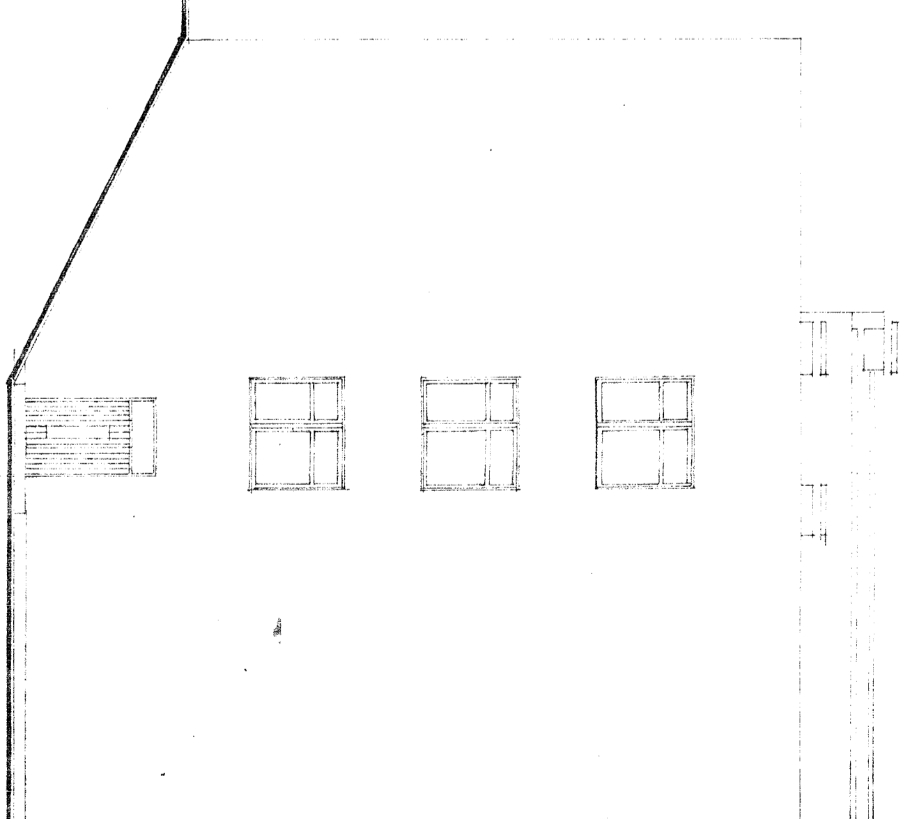
ELEWACJA WSCHODNIA 1:100
